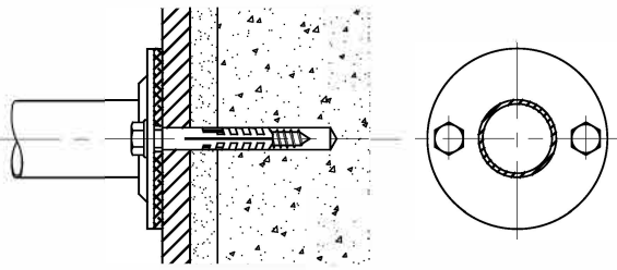
ДЕТАЛЬ А E= 1:3
